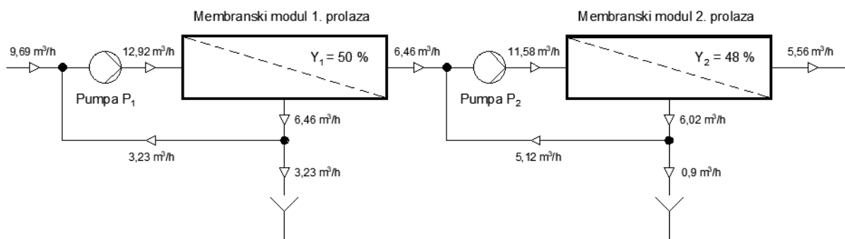
Slika 19. Shematski prikaz RO sustava
