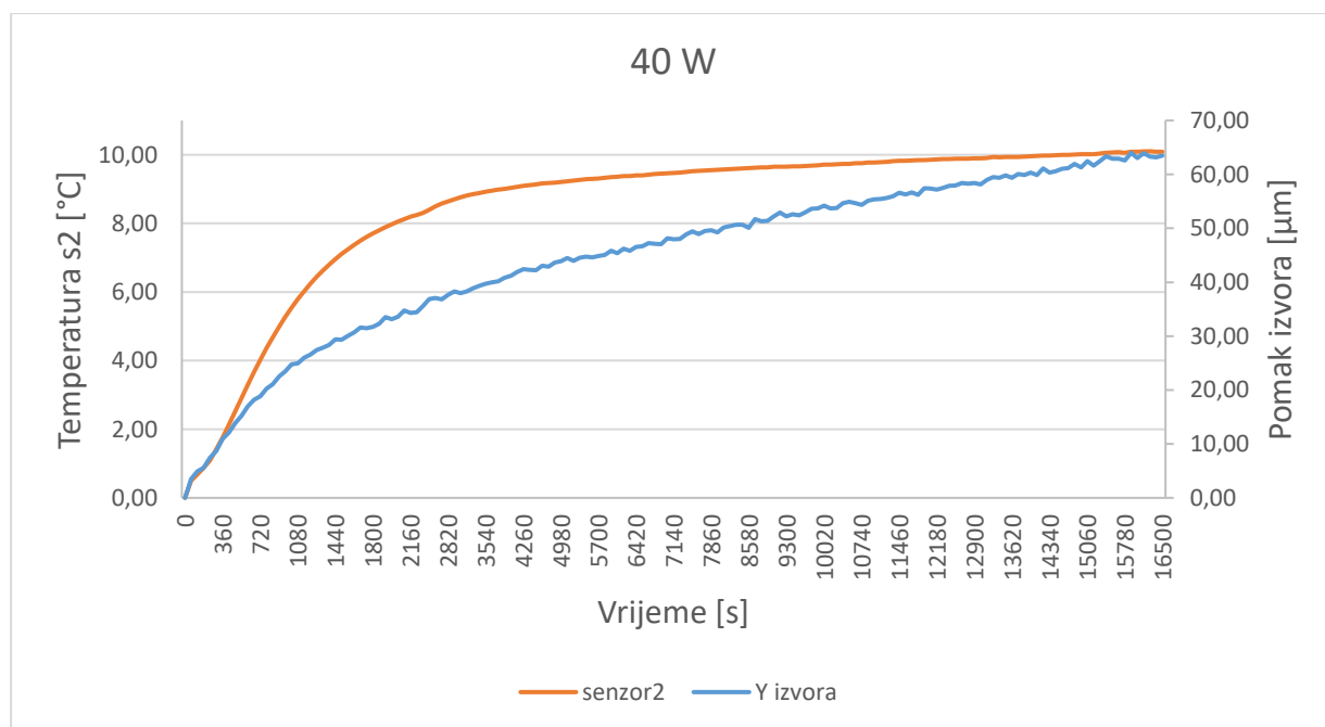
Slika 47 Usporedba promjene temperature senzora 2 i pomaka izvora po Y osi
