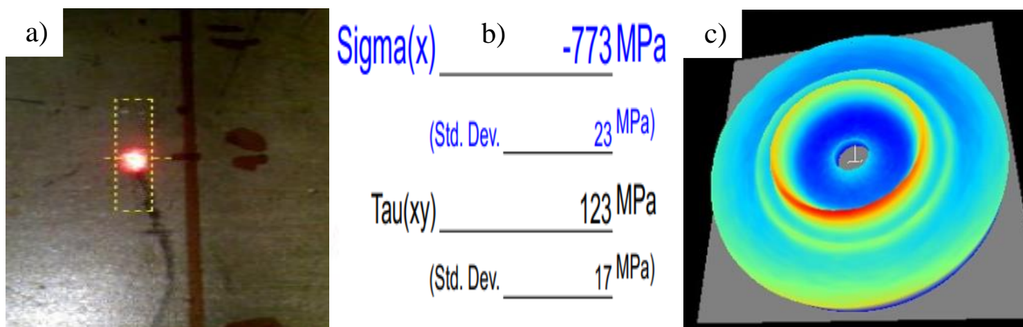
Slika 51. Prikaz: a) mjesta mjerenja kritične točke 10, b) iznosa napreznaja kritične točke 10. i c) pripadajući izgled Debye prstena
