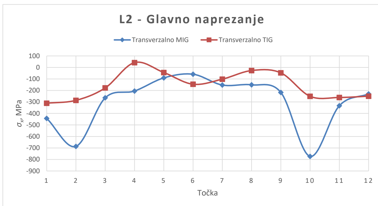
Slika 50. Usporedba glavnih transverzalnih napreznaja MIG i TIG uzorka na L2
