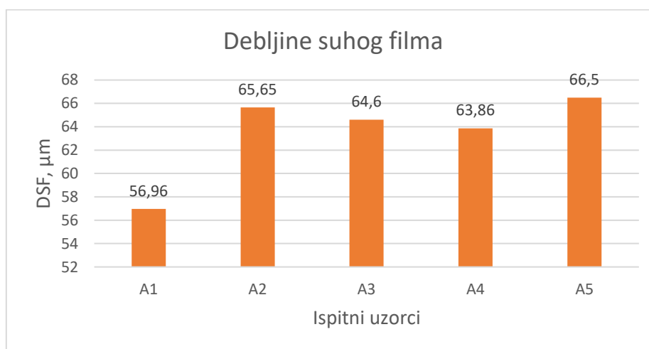
Slika 40. Debljine suhog filma ispitnih uzoraka s dva sloja premaza
