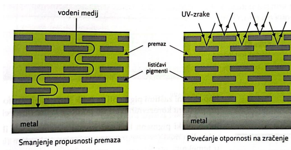
Slika 13. Učinak nepropusnih listićavih pigmenata u premazu [1]
