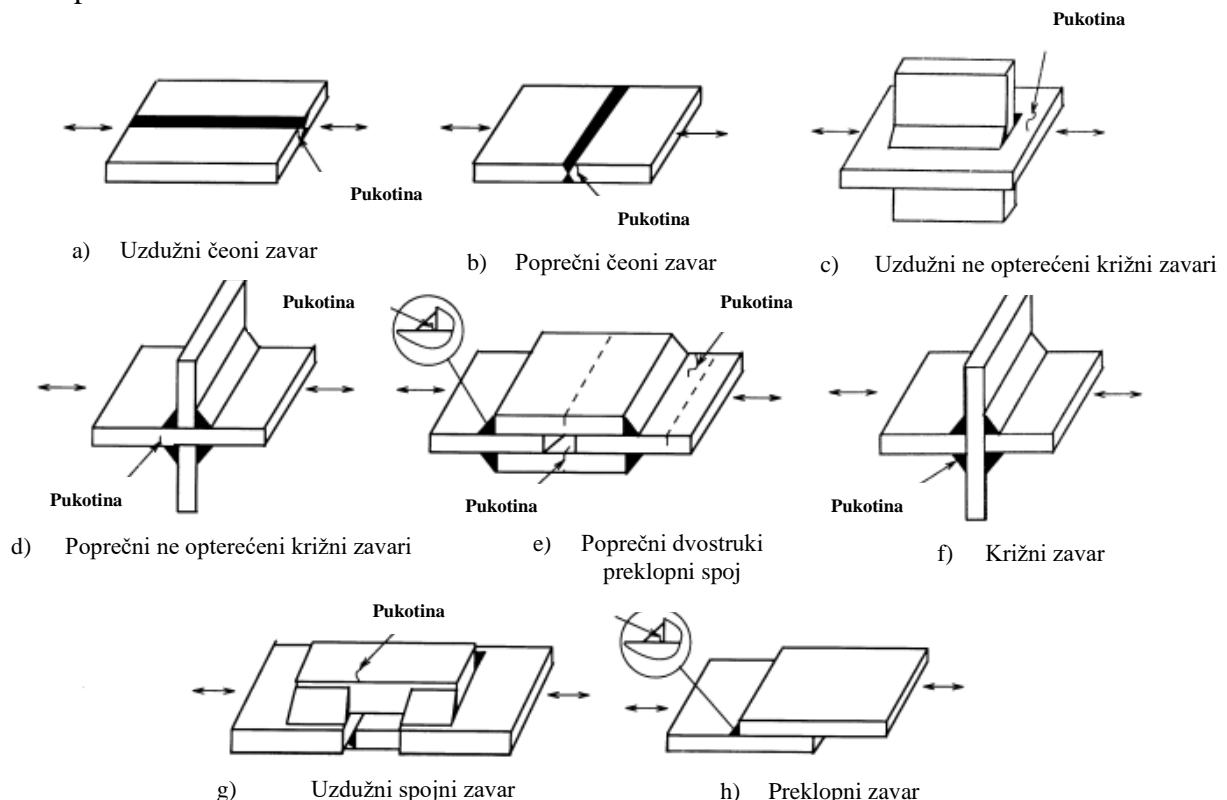
Slika 17. Detalji zavarenih dijelova aluminijskih legura sa označenim pukotinama [5]
