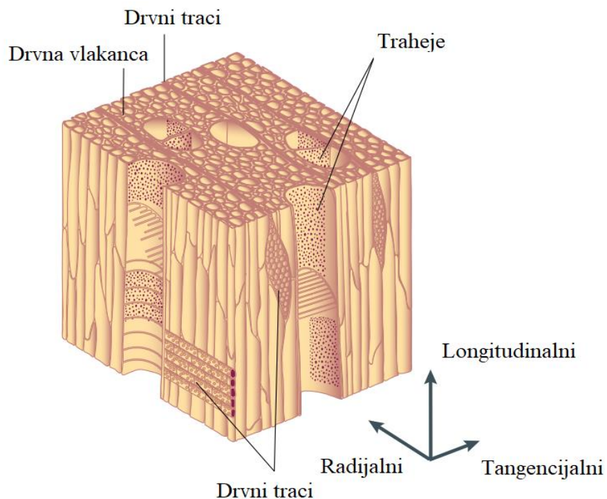
Slika 2.19 Mikrostruktura listača [1]
