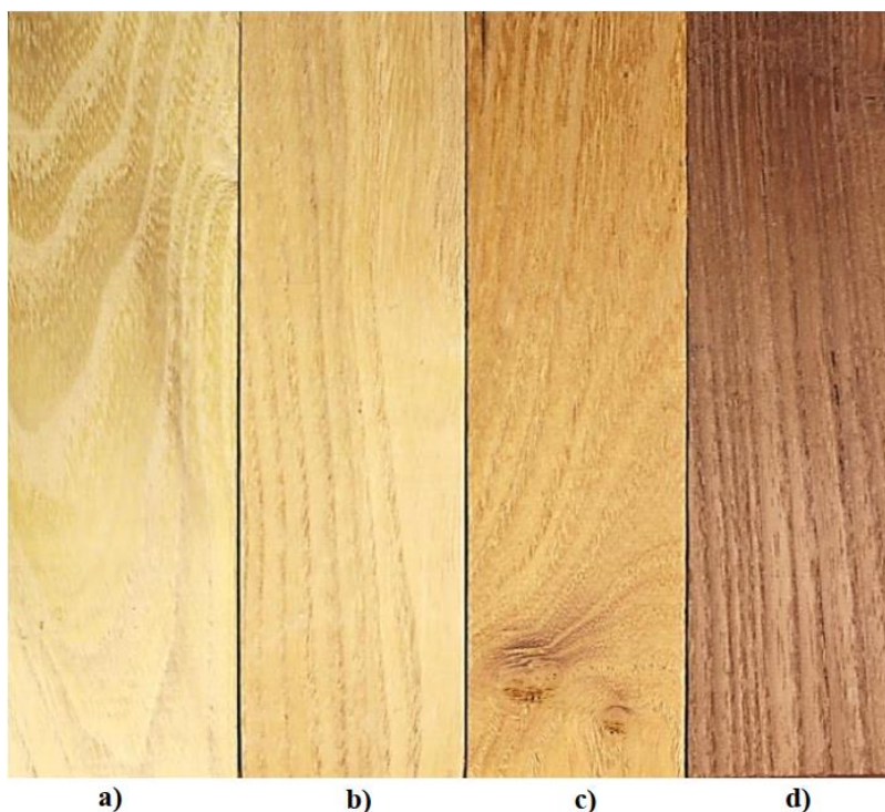
Slika 4.5 Tekstura drva bagrema prije i nakon toplinske obrade pri različitim parametrima a) prirodna boja, b) svijetlosmeđa boja, t = 5,5 h, T = 110 °C, c) sivkasto - smeđa boja, t = 6,5 h, T = 125 °C d) sivo - smeđa boja, t = 7,5 h, T = 135 °C [32]
