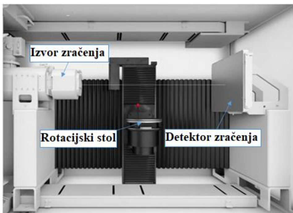
Slika 5.11 Dijelovi CT uređaja [35]
