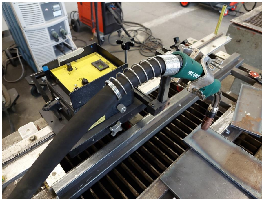
Slika 22. Modularni sustav za automatizirano zavarivanje MDS-1002 proizvođača Bug-O
