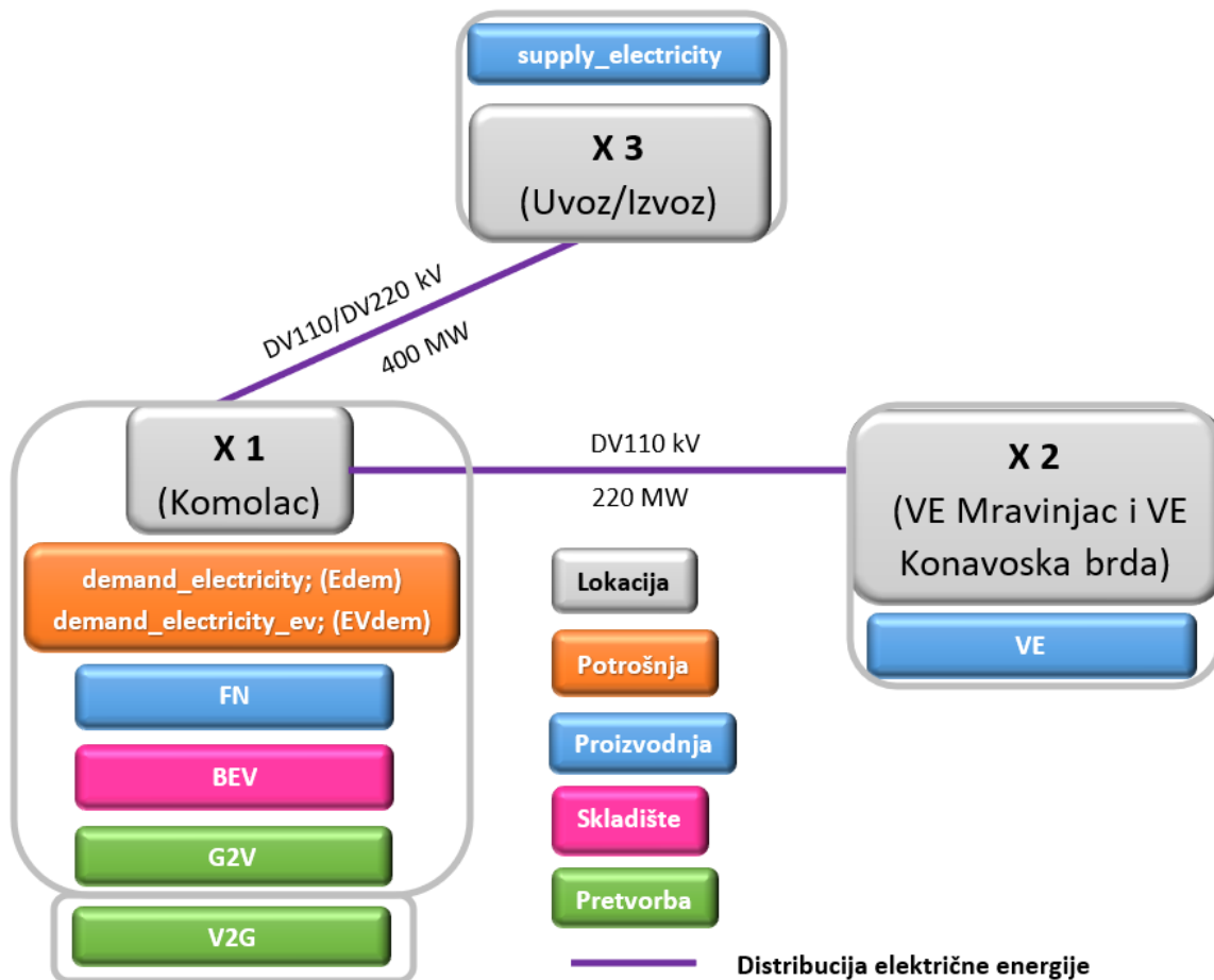
Slika 28. Model energetske sustava odabranog područja u programu Calliope prema scenariju S1
