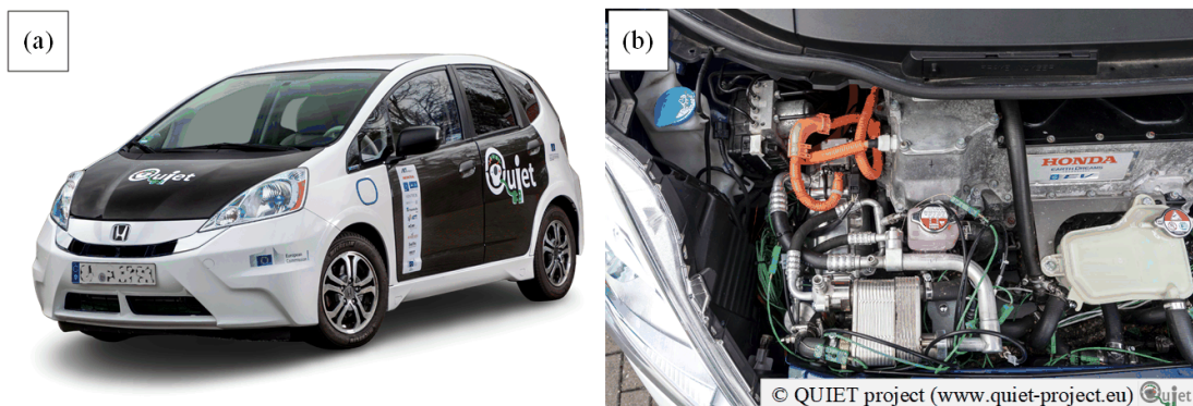
Slika 8-1. Eksperimentalno baterijsko električno vozilo (a) i ugrađeni HVAC sustav (b)
