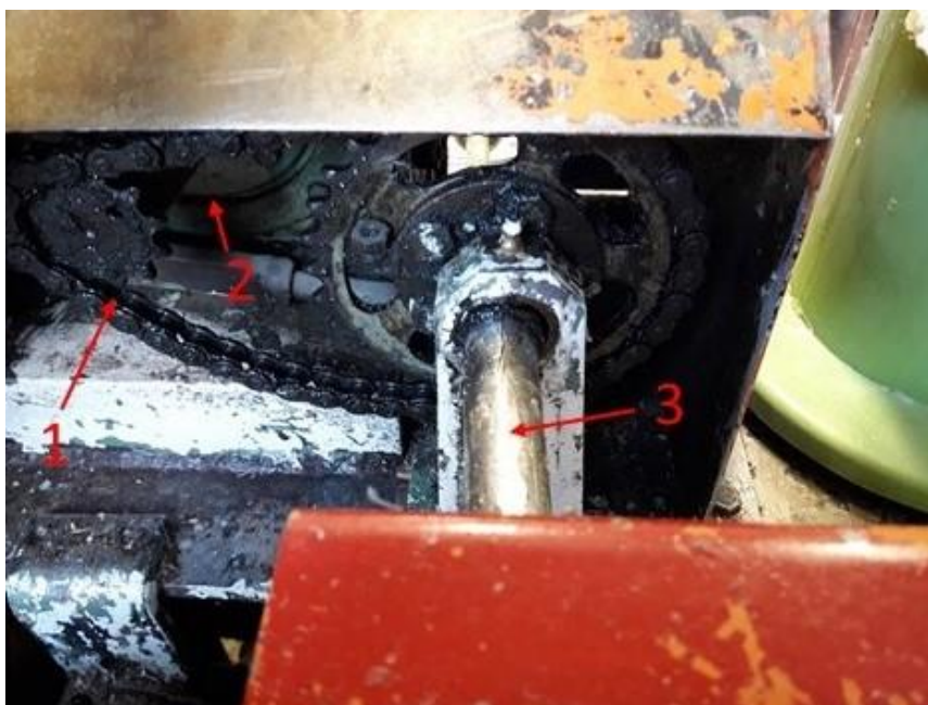
Slika 11. Sustav za okretanje predložaka (1 – lančani prijenos, 2 – prijenosnik snage, 3 – vratilo)
