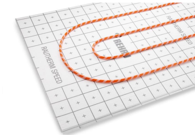
Slika 4-1. Rehau Tacker stiropor sustav podnog grijanja
