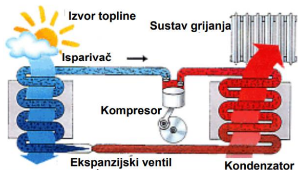
Slika 1-5. Shema ljevokretnog procesa [1]
