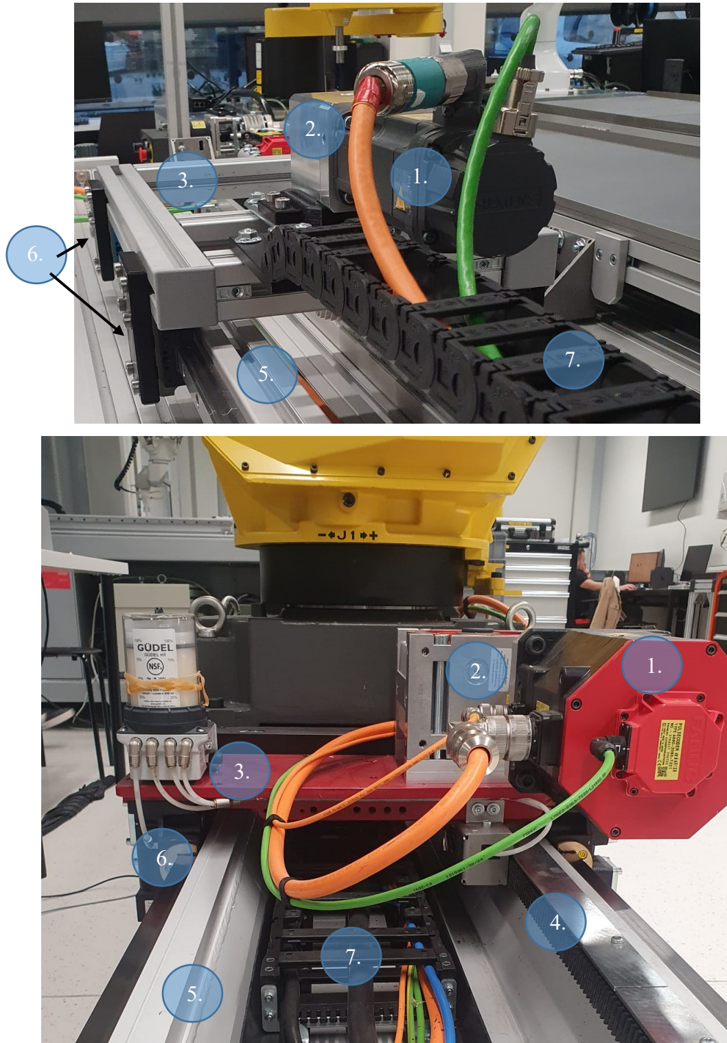
Slika 23. Usporedba s industrijskim rješenjem. 1. – motor, 2. – reductor, 3. – platforma, 4. – zupčasta letva, 5. – nosiva konstrukcija, 6. – vagoni na vodilicama, 7. – IGUS energy chain
