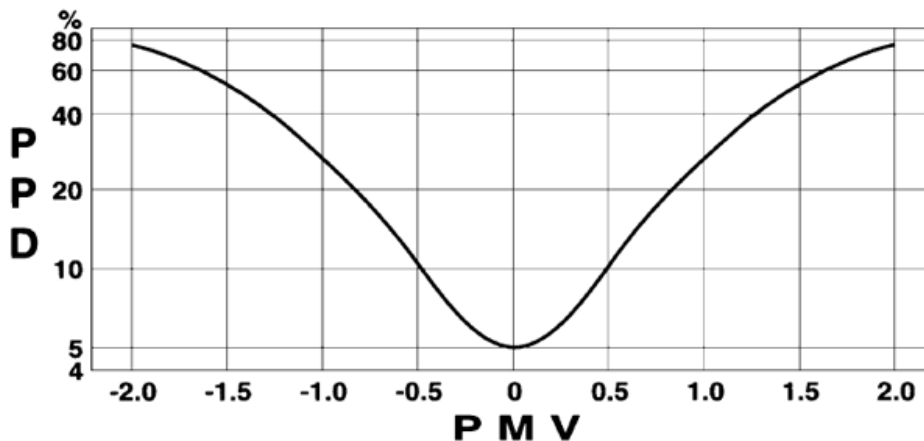
Dijagram 1. Odnos između PPD i PMV indeksa [4]
