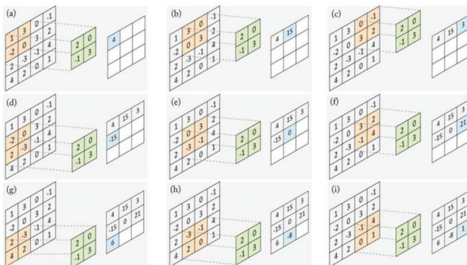
Slika 3.3 Konvolucija[11]
