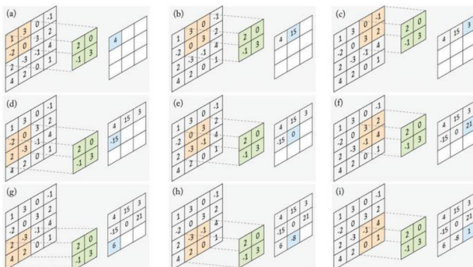
Slika 3.3 Konvolucija[11]
