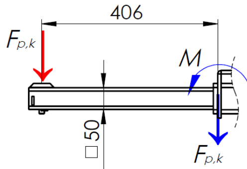
Slika 26. Konusni prihvrat prednjeg modula
