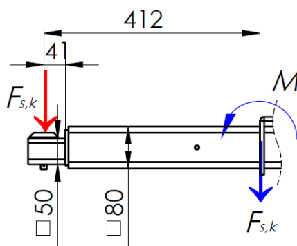
Slika 30. Konusni prihvat stražnjeg modula
