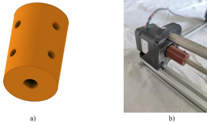
Slika 36. Spojka : a) 3D model spojke, b) prikaz montaže 3D ispisanog spojke i vratila koračnog motora
