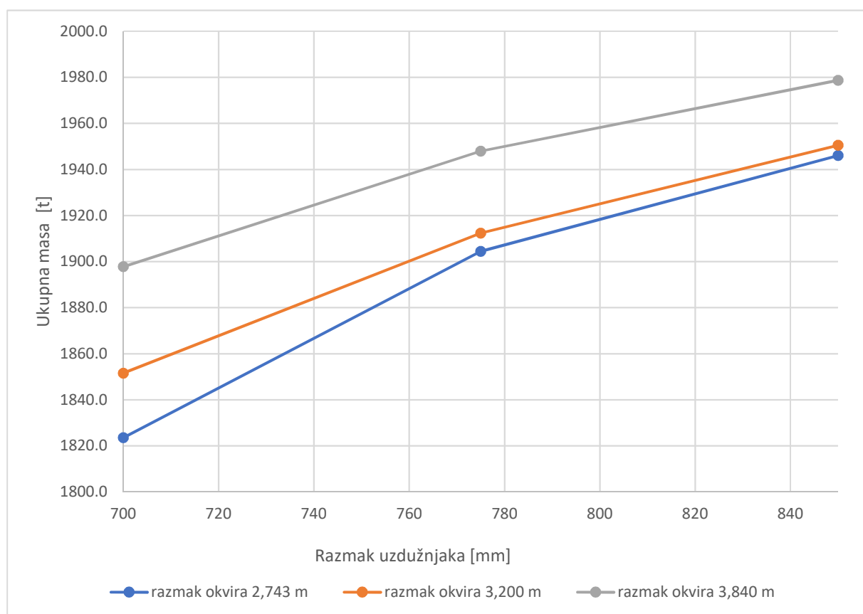
Slika 22. Ukupna masa – MODEL B
