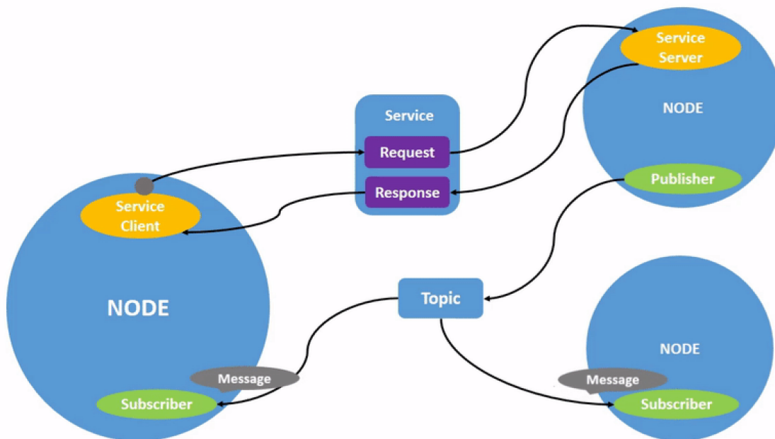
Slika 3.1 Jednostavan prikaz graf arhitekture ROS-a [16]
