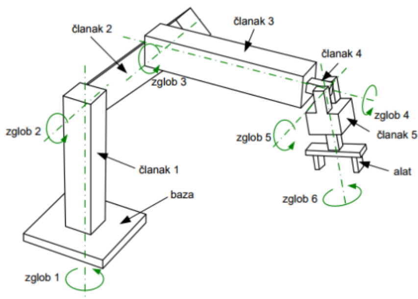
Slika 4. Prikaz dijelova robota manipulatora [6]
