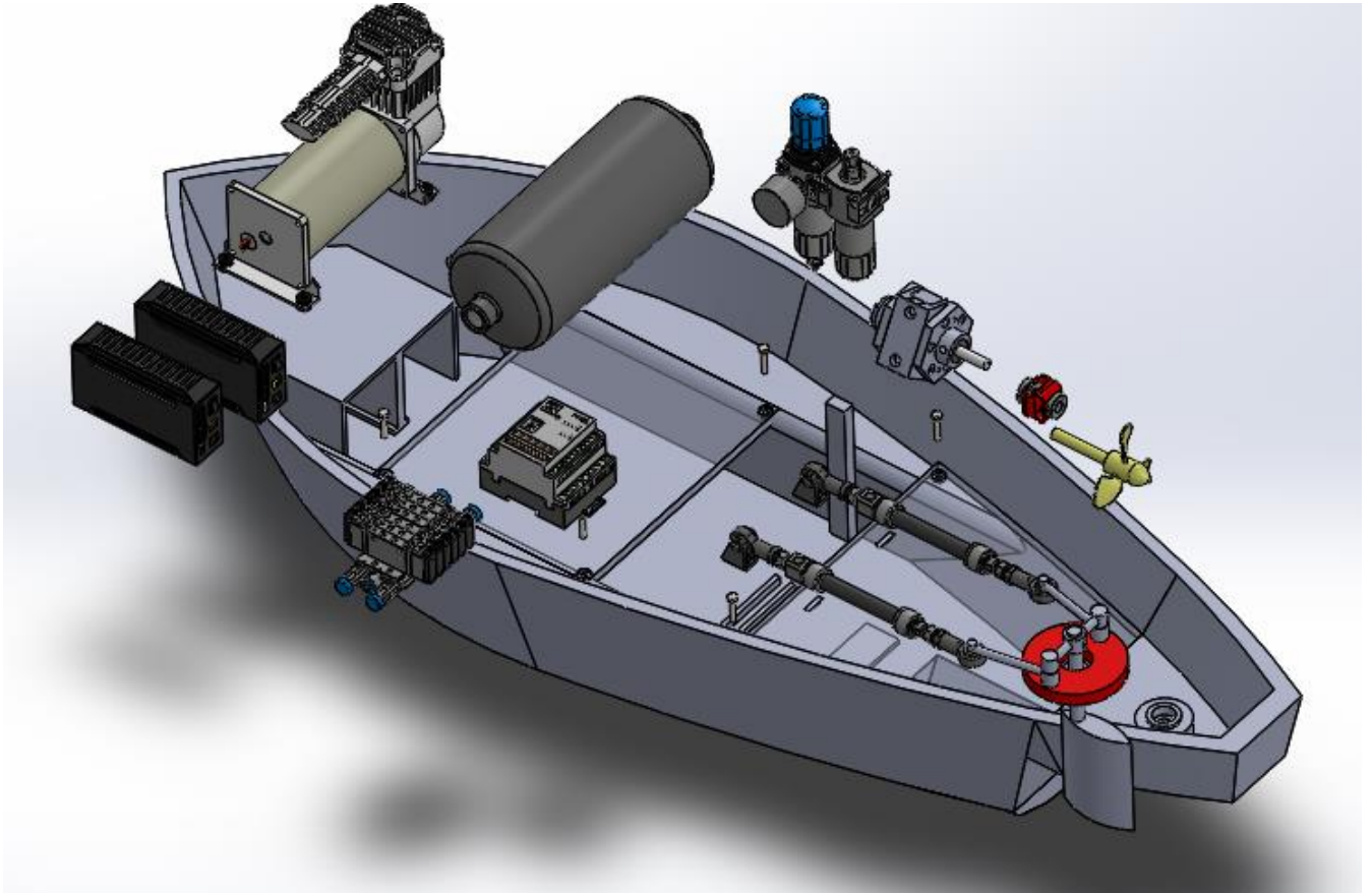
Slika 3.14. Eksplozirani pogled na model brodice
