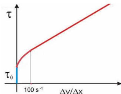
Slika 2.2 Odnos smičnog napreznja i gradijenta brzine kod krvi [6]
