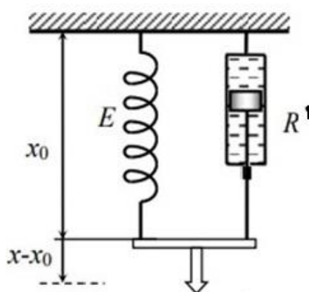
Slika 2.4 Kelvin – Voigtov model
