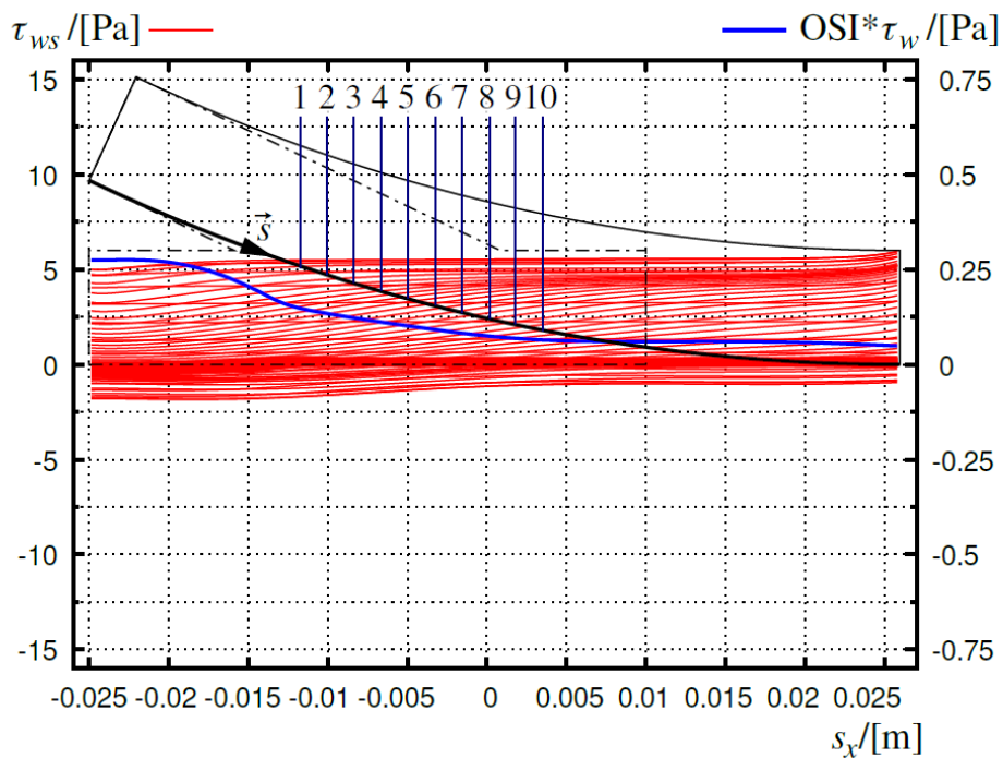
Slika 6.9 Grafički prikaz anvelope smičnog naprežanja i OSI \cdot \tau_w duž donje izvodnice – slučaj A
