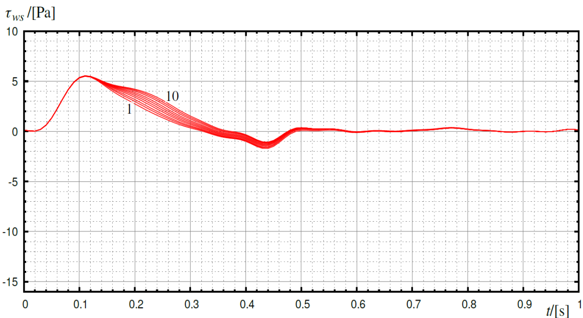
Slika 6.10 Grafički prikaz vremenske promjene smičnog naprežanja u odabranim točkama duž donje izvodnice – slučaj A
