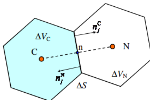
Slika 4.2 Kontrolni volumen u interakciji s okolinom
