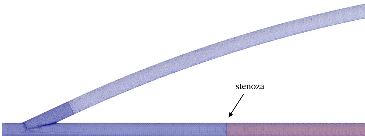
Slika 5.3 Prikaz položaja stenozne u odnosu na ulaznu račvu u slučaju B
