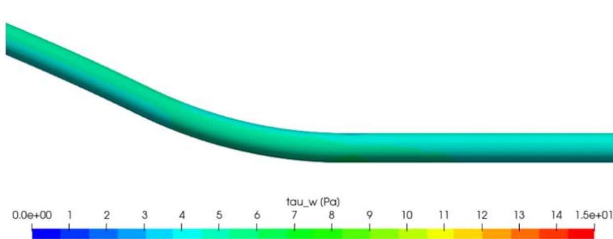
Slika 6.5 Maksimalno smično naprezanje na izlazu iz premosnice – slučaj A
