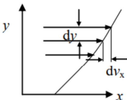
Slika 2.1 Gradijent brzine
