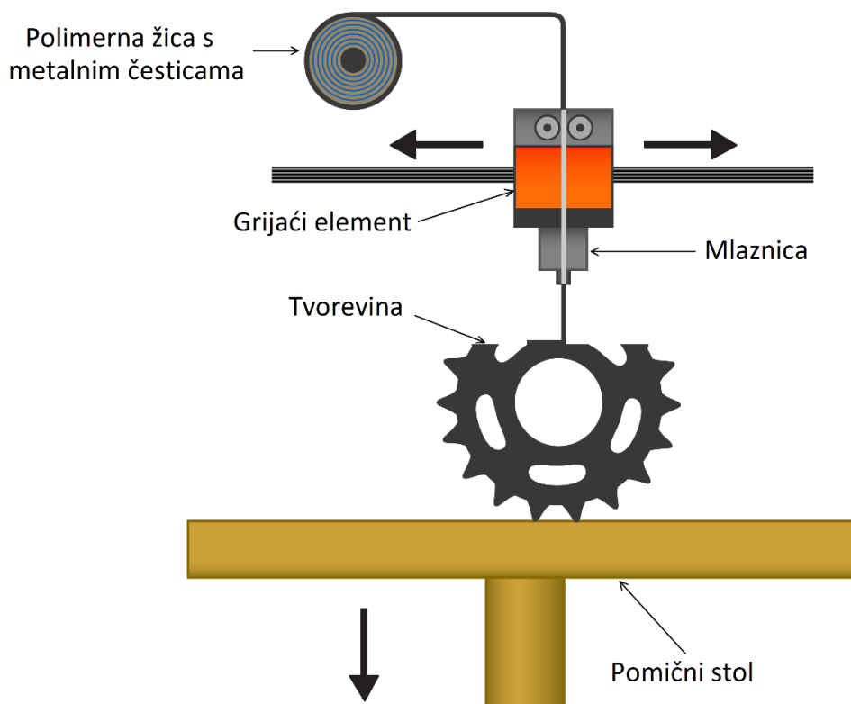
Slika 2.12. Postupak MME [20]
