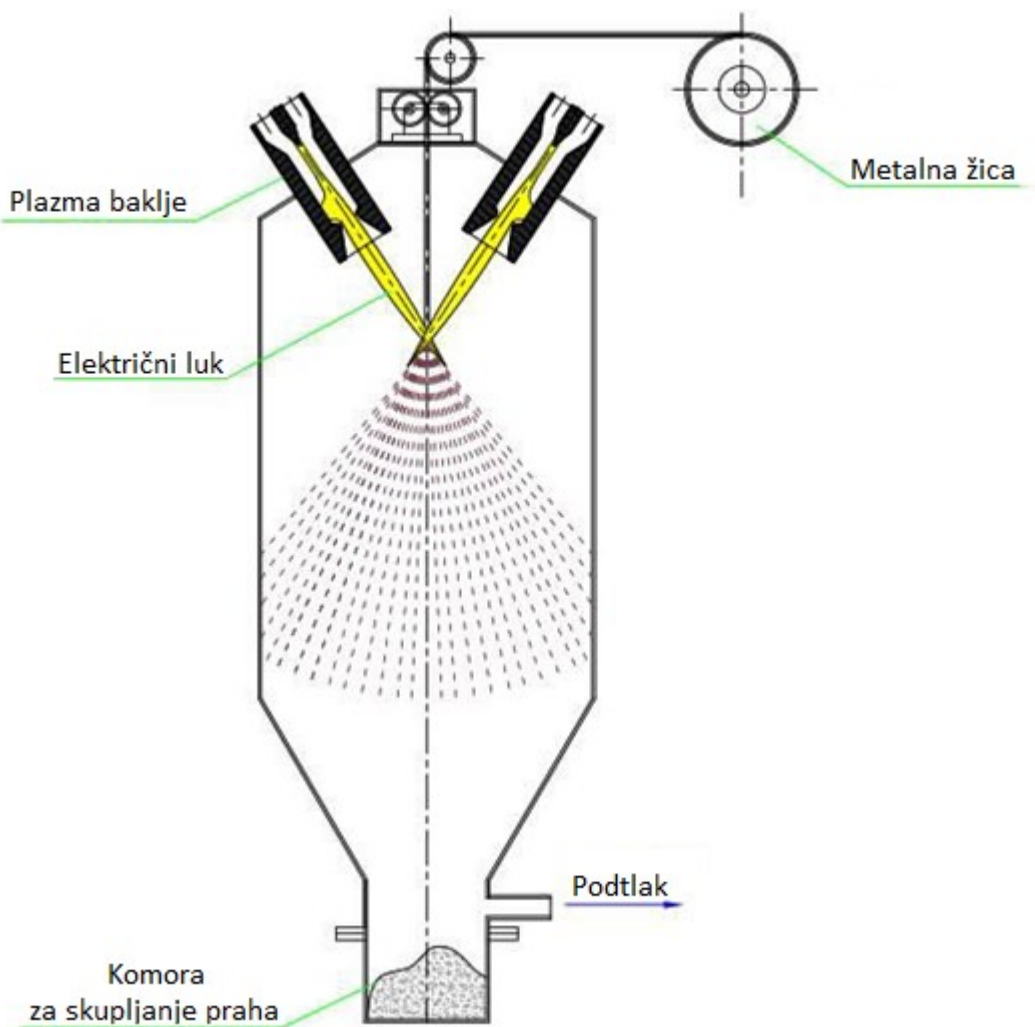
Slika 3.2 Atomizacija plazmom [33]
