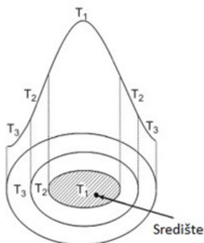
Slika 3.4. Raspodjela temperature u laserskoj zruci [36]
