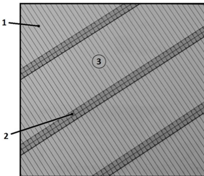
Slika 4.2. "NoPattern" strategija skeniranja [101]
