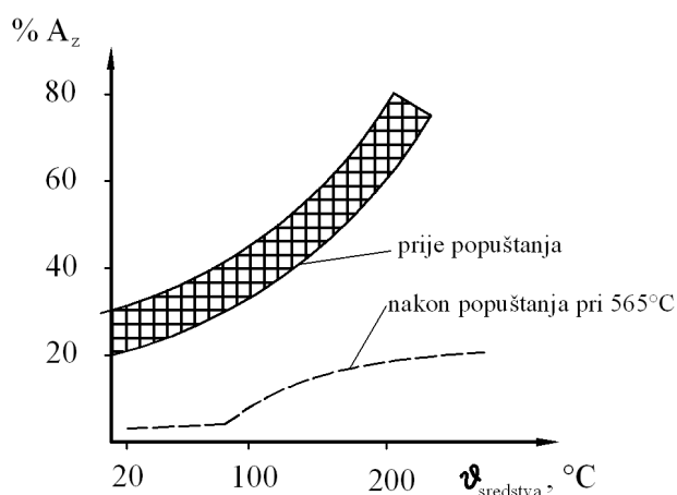
Slika 2.7. Utjecaj temperature sredstva za gašenje na udjele zaostalog austenita čelika S 6-5-2 (C7680) [1]
