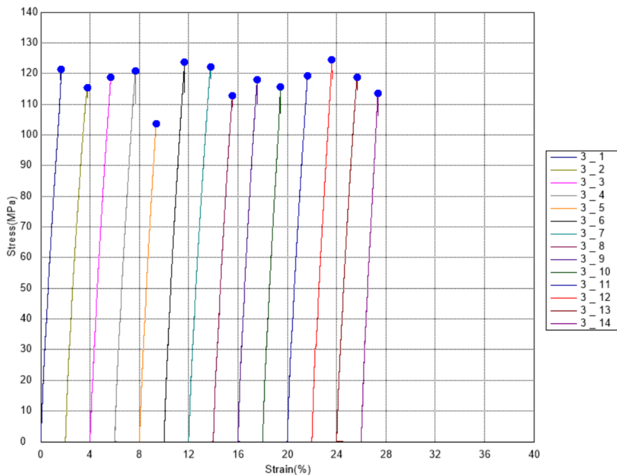
Slika 12. Graf naprezanje-istezanje za EP/6lan
