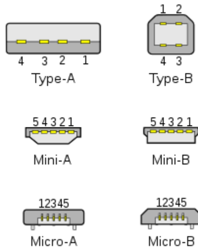
Slika 6. USB standardi
