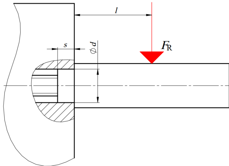
Slika 39. Opterećenje ručke
