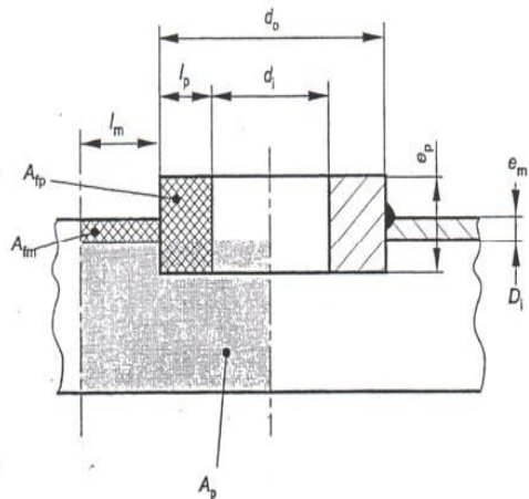
Slika 7. Ojačanje umetcima
