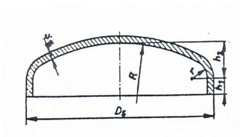
Slika 3. Ispupčena puna podnica
