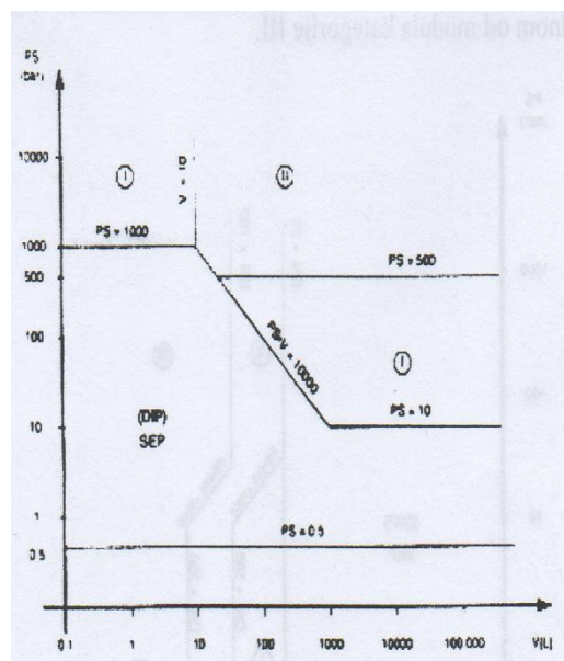
Dijagram 4. Posude za kapljvine grupe 2
