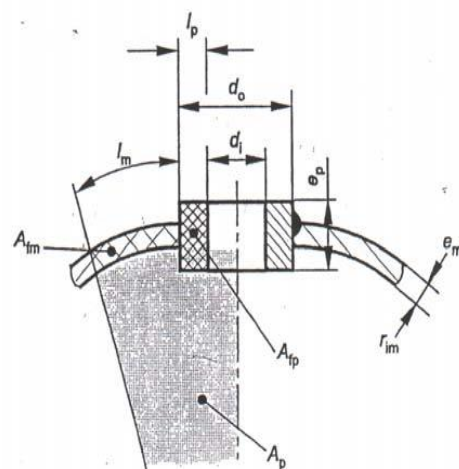
Slika 8. Ojačanje umetcima-poprečni presjek
