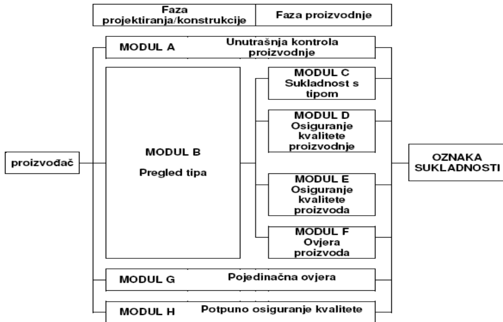
Slika 2. Shema modula za ocjenu sukladnosti
