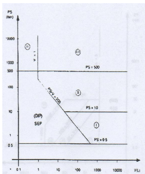
Dijagram 3. Posude za kapljvine grupe 1
