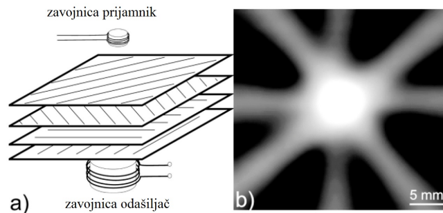
Slika 18: Magnetsko polje u multidirekcijskom CFRP uzorku: a) mjerenje magnetskog polja, b) prikaz z komponente magnetskog polja u skeniranom području [6]
