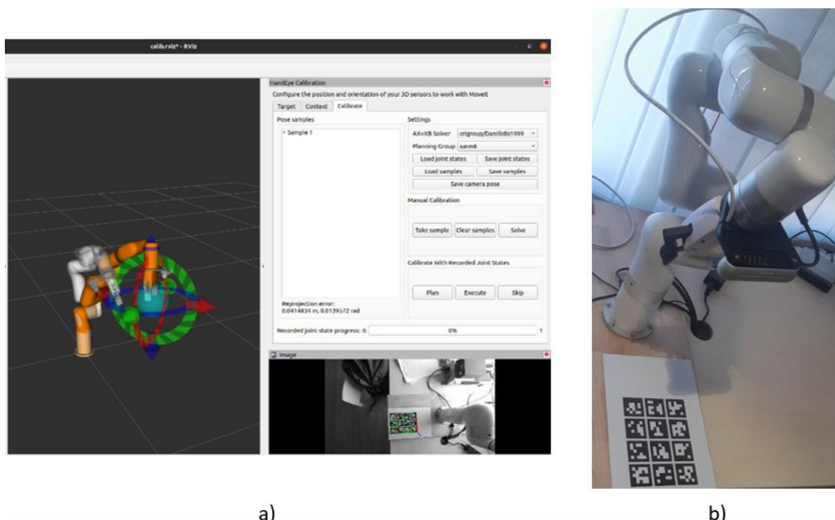
Slika 3.9 a) Kalibracijski alat unutar RViz-a, b) Prikaz robotske ruke prilikom kalibracije
