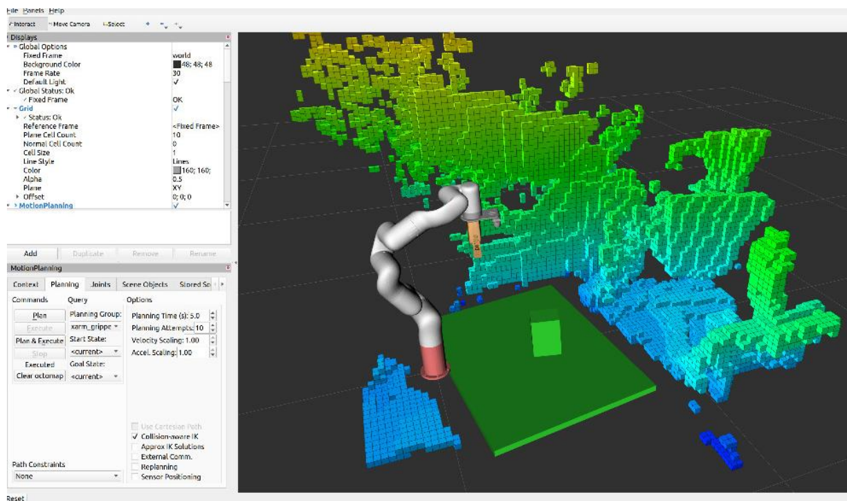
Slika 3.21 Prikaz dodanih geometrijskih primitiva u ROS okolinu kao objekti za manipulaciju
