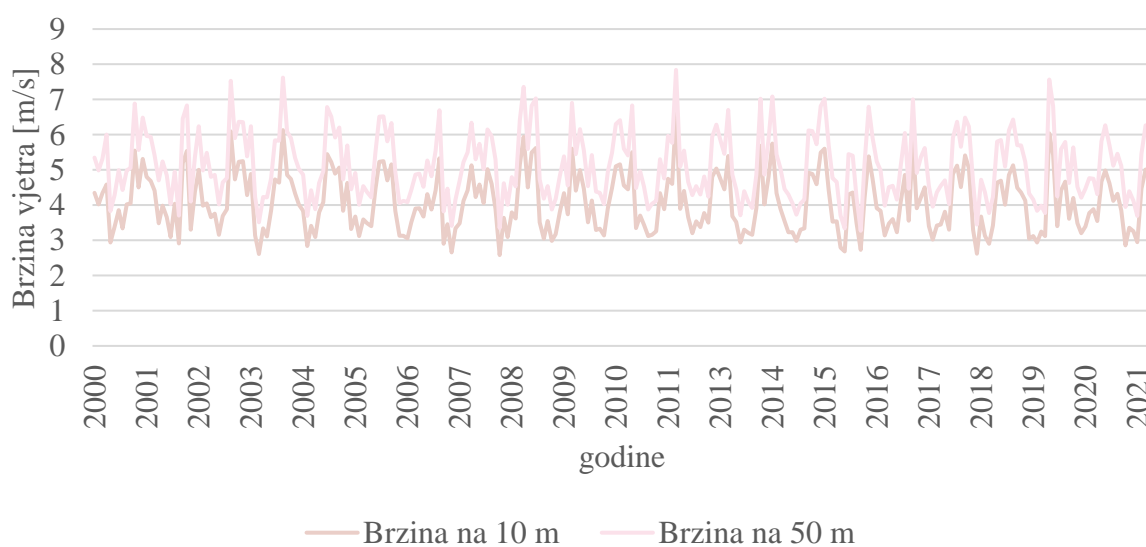
Slika 51. Brzina vjetra u Splitu
