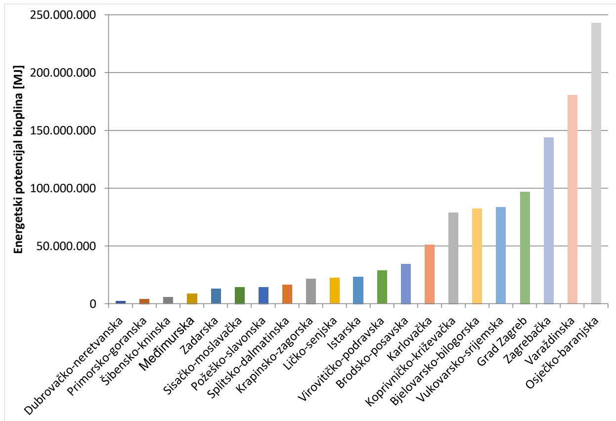
Slika 21. Energetski potencijal bioplina iz stočarske proizvodnje po županijama
