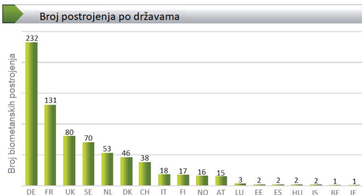
Slika 3. Bioplinska postrojenja po državama [27]
