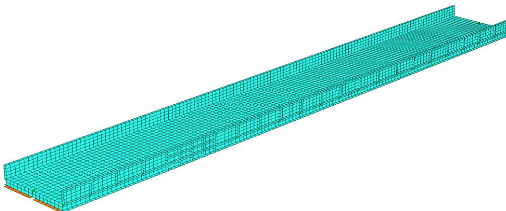
Slika 9. Strukturni model rampe varijante 2 (pogled s gornje strane)
