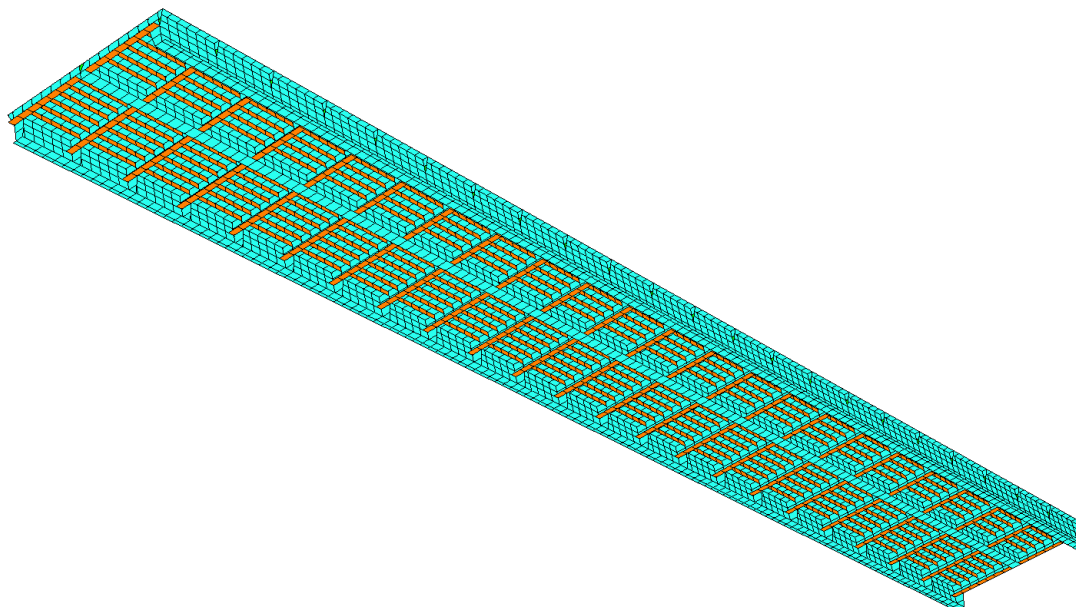
Slika 8. Strukturni model rampe varijante 1 (pogled s donje strane)
