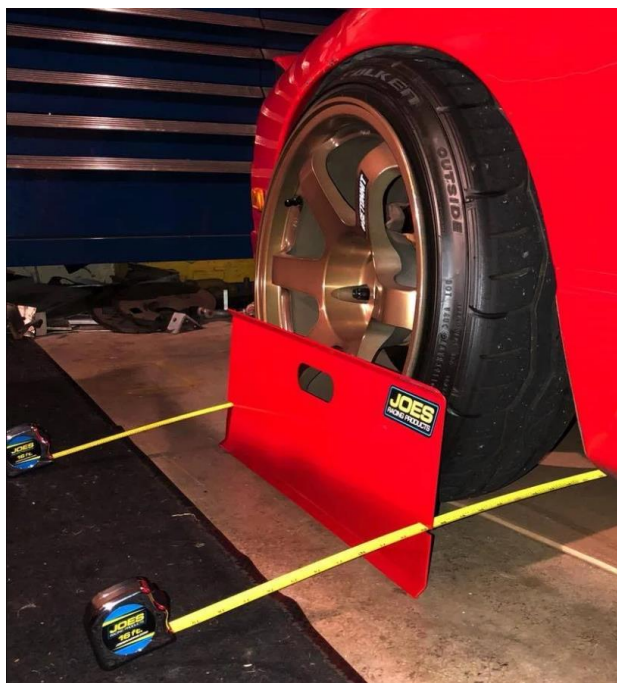
Slika 4.7. Ploče za mjerenje usmjerenosti kotača [12]
