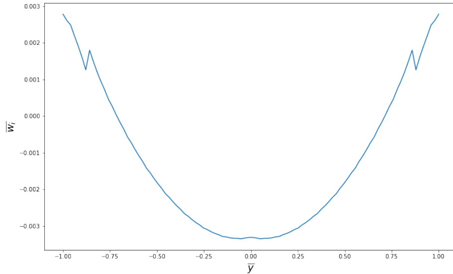
Slika 5.25: Inducirana brzina bez otklona upravljačkih površina
