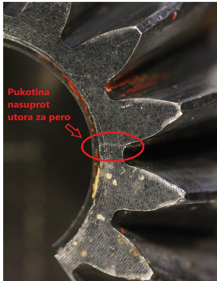
Slika 41. Pukotina nasuprot utora za pero-odozgo
