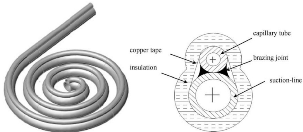
Slika 40 Izometrijski prikaz i presjek dijabatske kapilarne [28]
