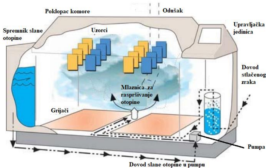
Slika 29. Slana komora [29]
