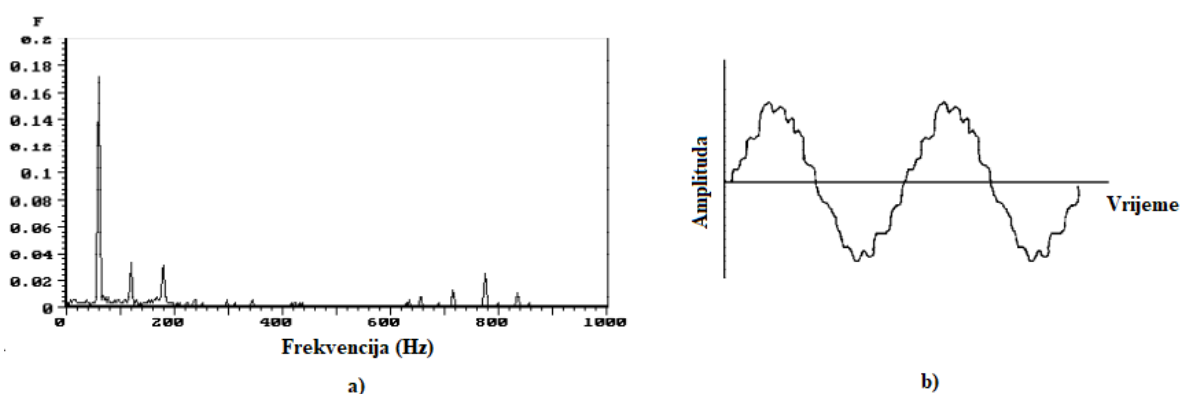
Slika 54. a) Spektra fourierovih transformacija, b) Snimljeni signal [37]
