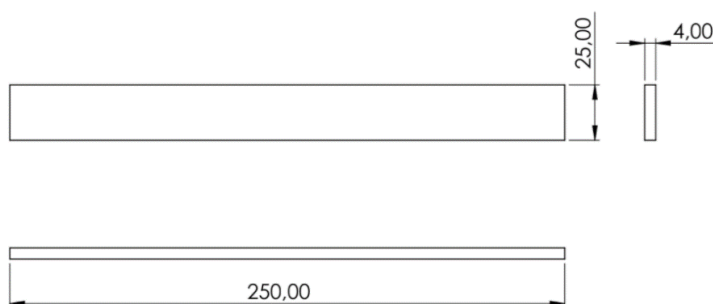
Slika 23. Pramodel za ispitivanje rastezних svojstava
