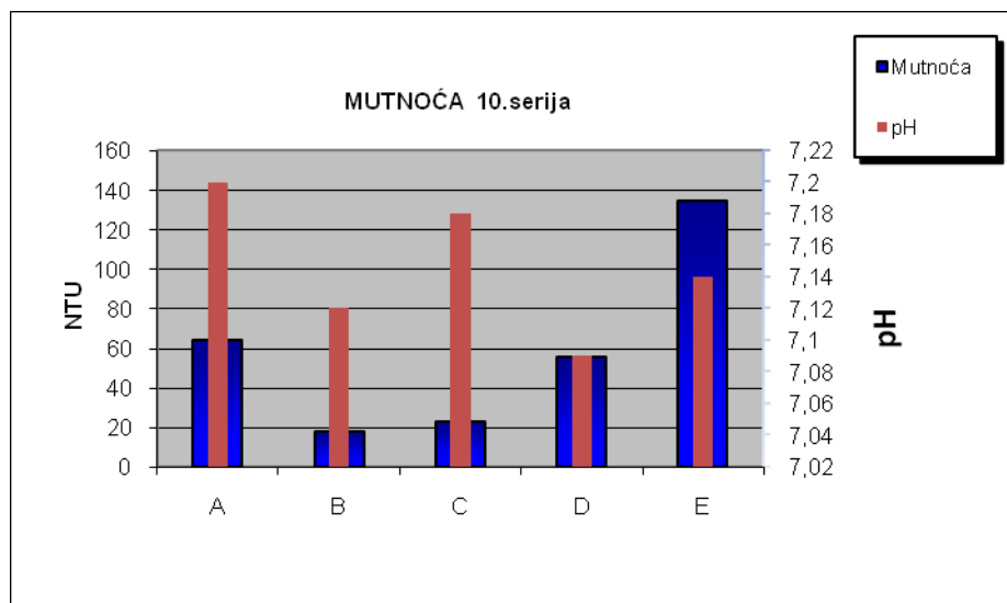
Dijagram 19. Prikaz mutnoće i pH-vrijednosti pri temperaturi =24^{20,5} \text{ }^{\circ}\text{C}
