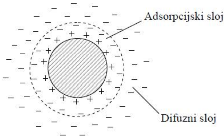
Slika 2. Shematski prikaz strukture micela, prema [2]
