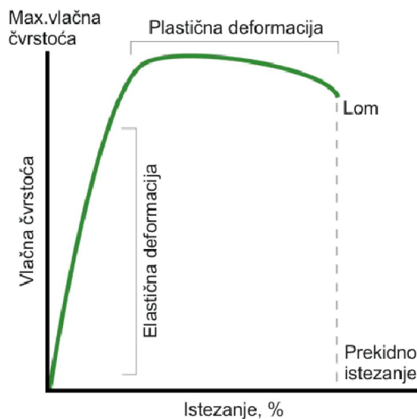
Slika 2 Svojstva materijala [1]
