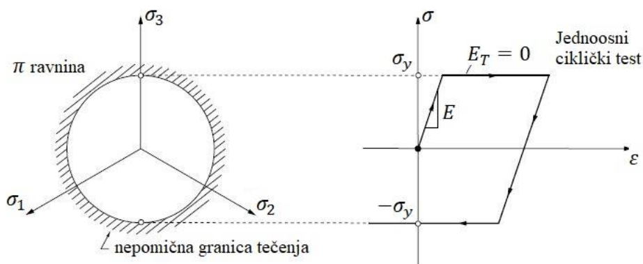
Slika 11 Idealna plastičnost. Prikaz jednoosnog cikličkog testa i granice tečenja u \pi ravnini [4]
