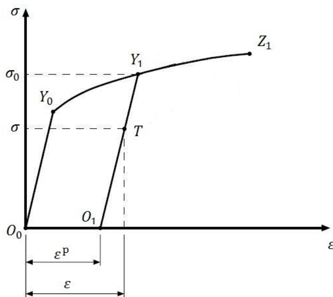
Slika 5 Shematski dijagram ovisnosti napreznja i deformacije za jednoosni vlačni test
