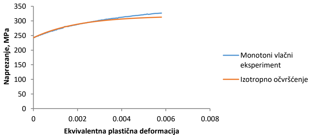
Slika 38 Model izotropnog očvršćenja i monotoni vlačni eksperiment za gustoću 6,8 \text{ g/cm}^3
