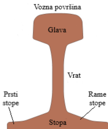
Slika 10. Dijelovi tračnice [20]
