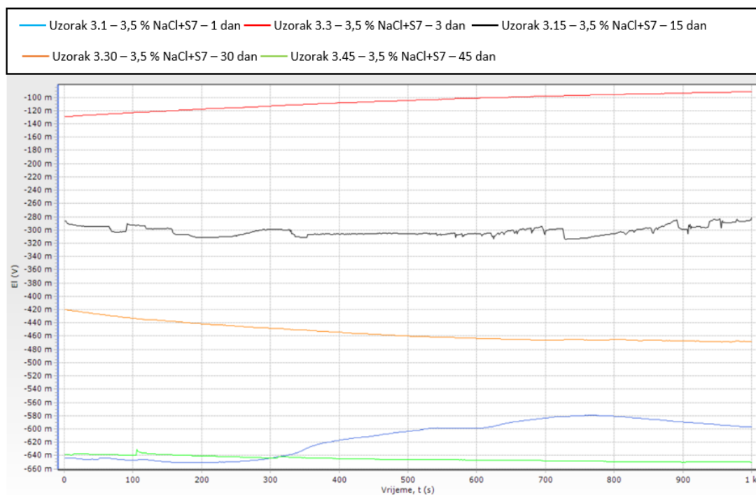
Slika 18. Usporedni dijagram korozijskog potencijala u 3,5 % NaCl s dodatkom S7
