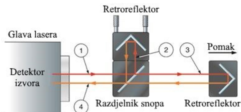
Slika 14. Prikaz primjene koncepta laserske interferetrije [33]
