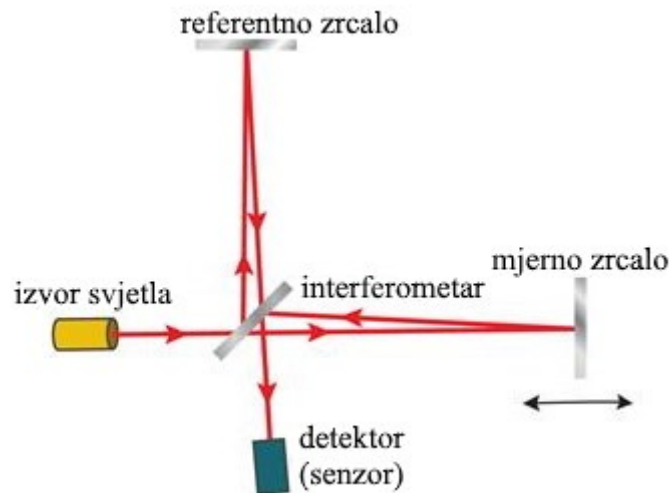
Slika 13. Osnovni koncept laserske interferetrije [33]
