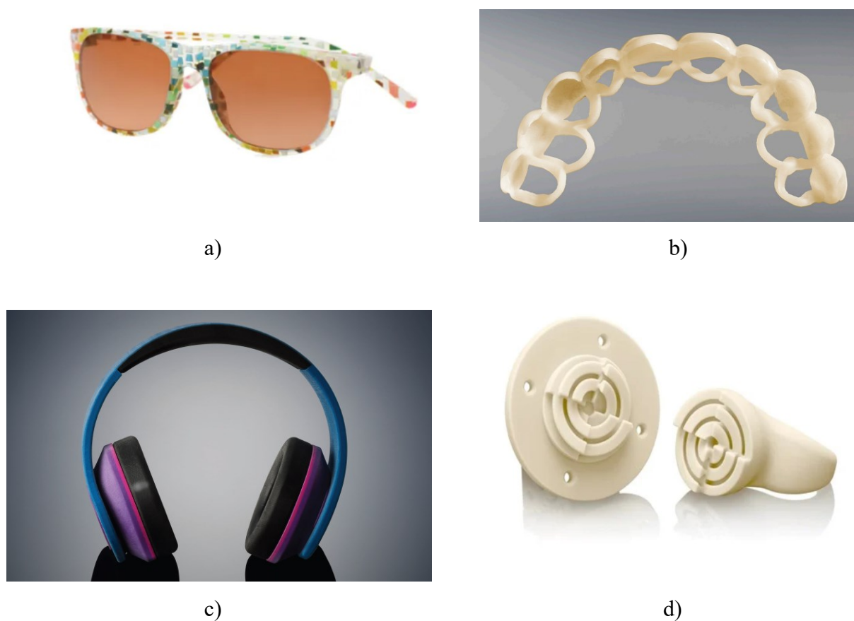
Slika 4.2. Primjeri proizvoda izrađenih postupkom PolyJet: a) VeroFlex okvir sunčanih naočala, b) VeroGlaze uzorak zubala, c) Tango jastučići na slušalicama, d) Digital ABS Plus model [14]
