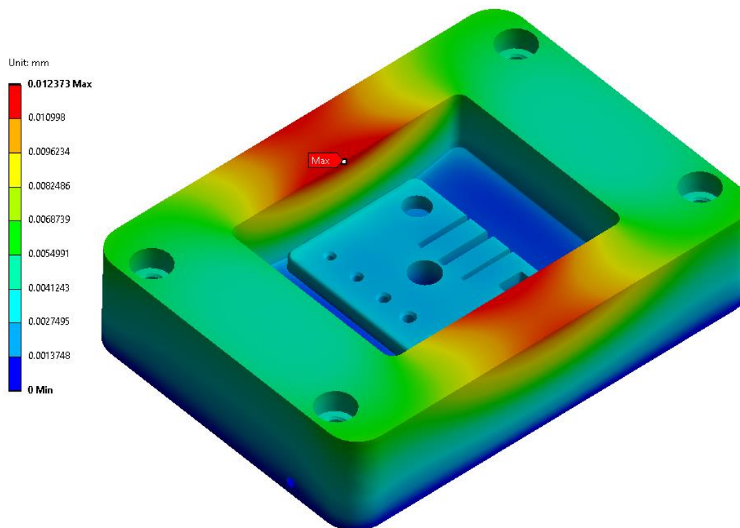
Slika 6. 33. Ukupna deformacija čelične matrice
