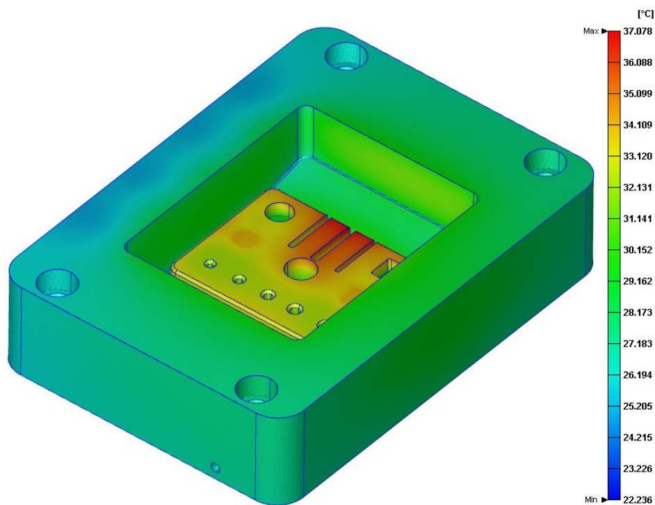
Slika 6. 20. Raspodjela temperatura na čeličnoj matrici
