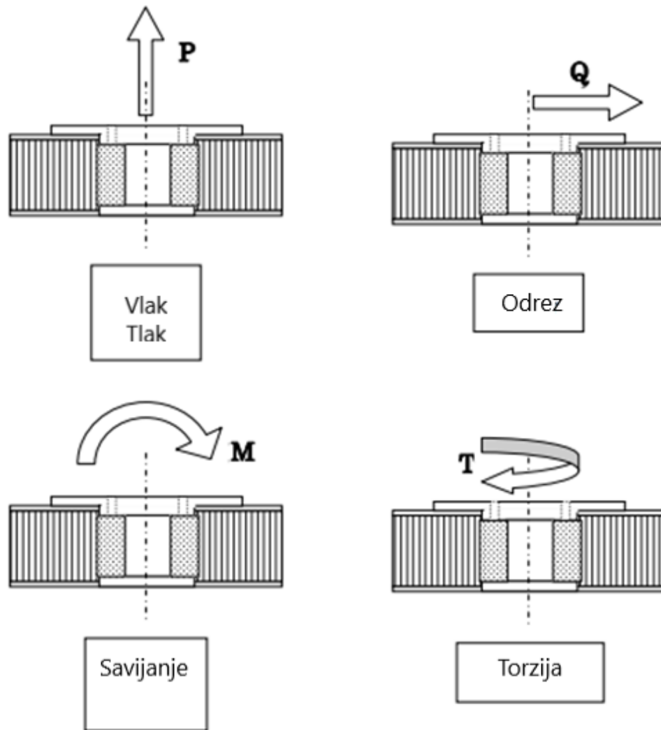
Slika 5.1. Vrste opterećenja umetaka [18]
