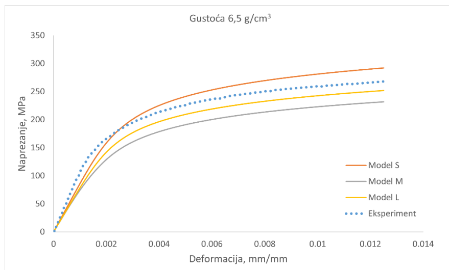
Slika 8.9 Dijagram normalno naprežanje u smjeru osi x -deformacija za gustoću 6,5 g/cm 3 za elastoplastično ponašanje materijala
