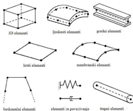
Slika 5.1 Osnovni konačni elementi [15]
